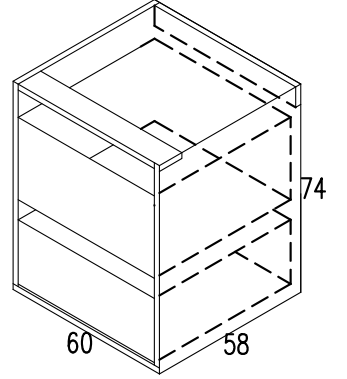
standart alt 2 çekmeceli dolap
