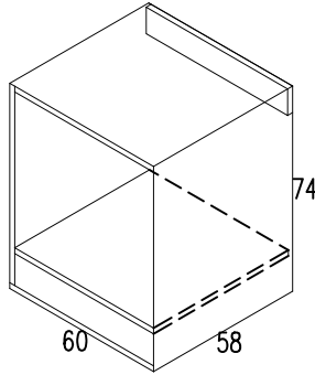
standart fırın dolabı
