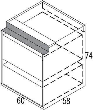
standart 2 çekemceli alt dolap
