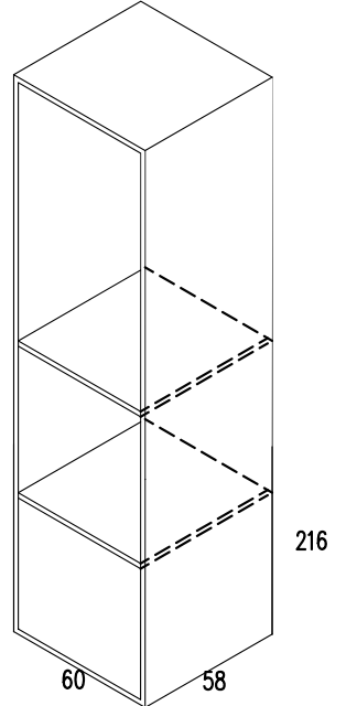
ankastre fırın dolabı
