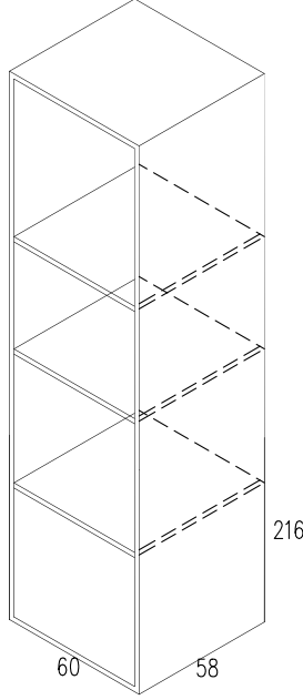
ankastre mikrodalga + fırın dolabı
